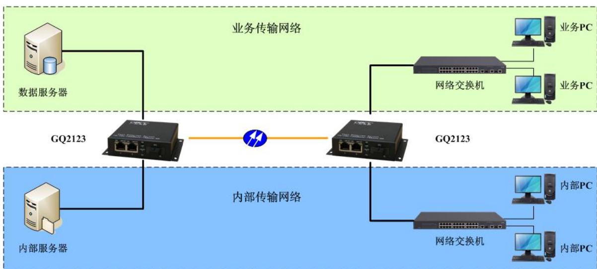
光纤组网方案图
