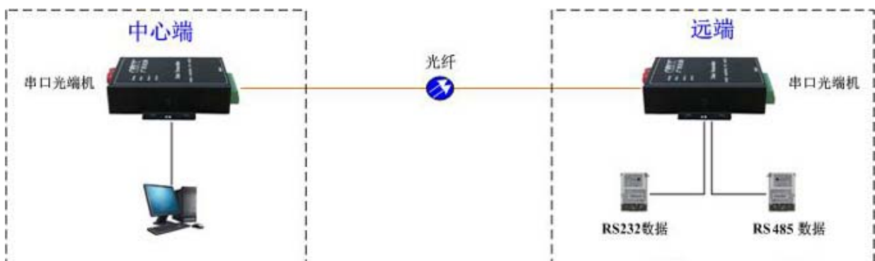
光纤点对点组网
